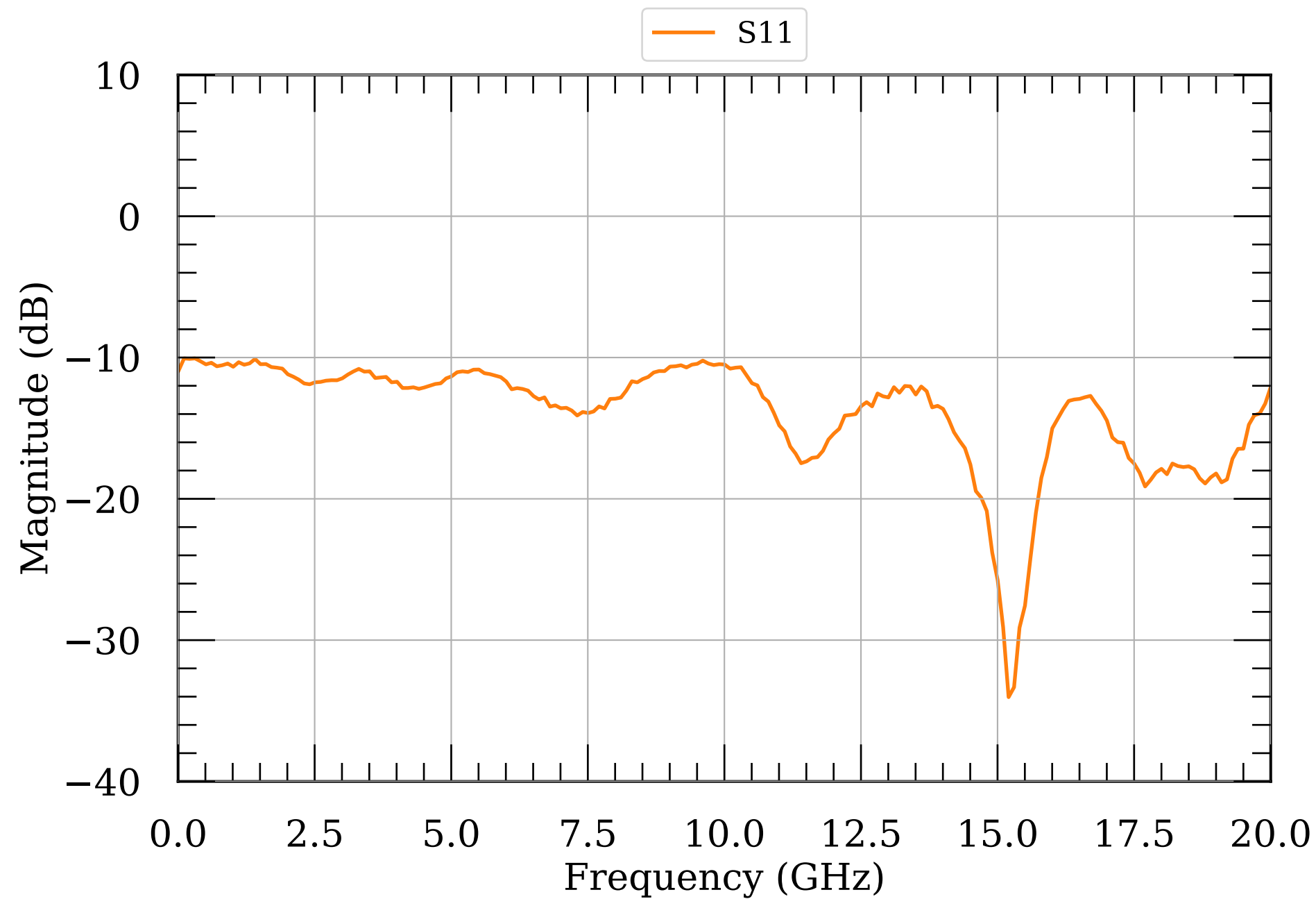
LNA S-params module096
